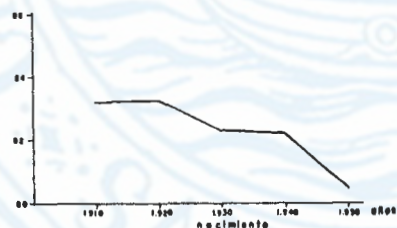
Fig. 3 Evolución del I. CEFALICO en una población adulta
