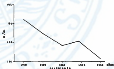
Fig. 5 Anchura Cefálica máxima
