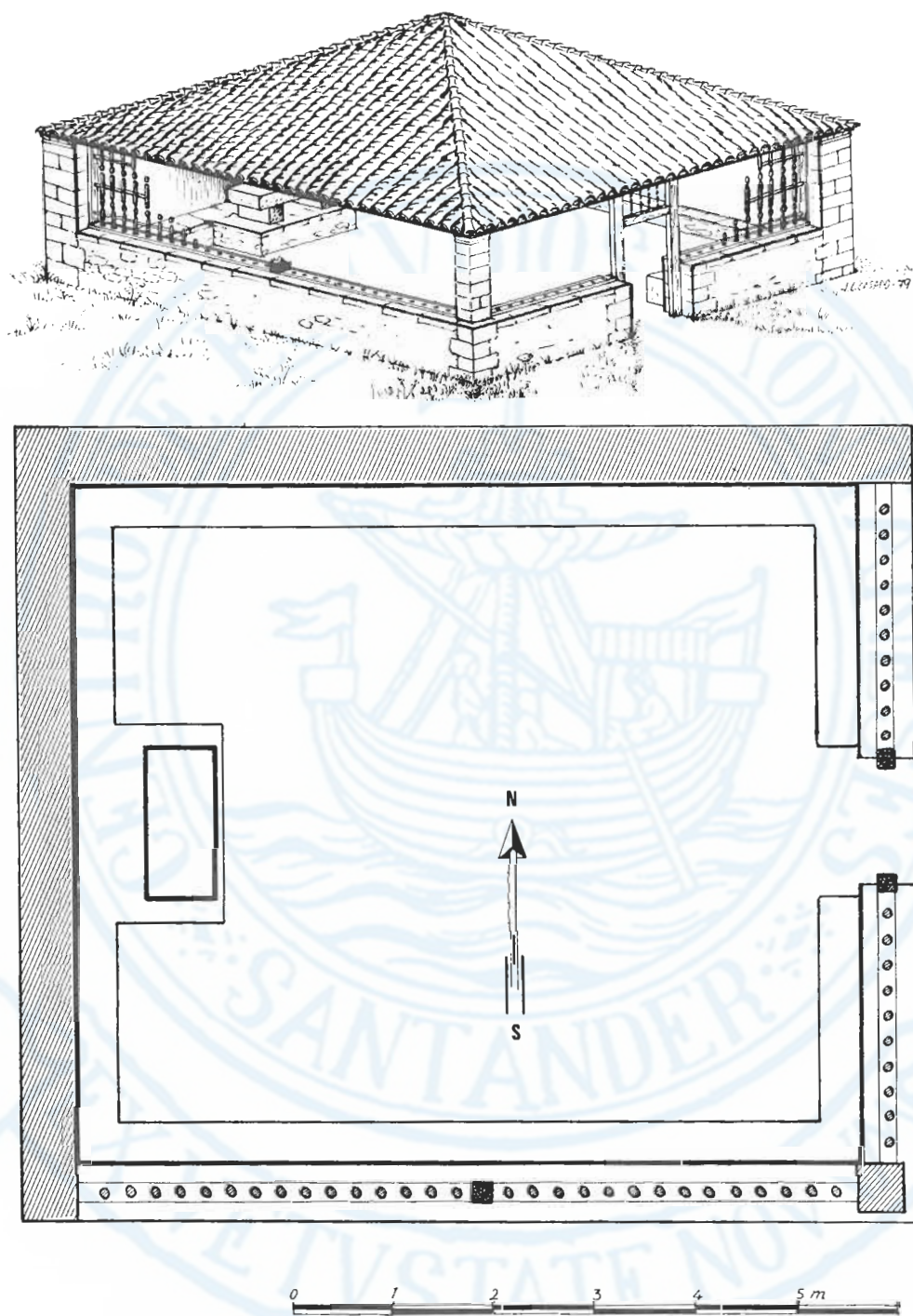
Figura 1.—Proyección isométrica y planta de la Casa de Juntas de los Nueve Valles, en Puente San Miguel, utilizada por la Provincia de Cantabria para sus Asambleas Generales.
