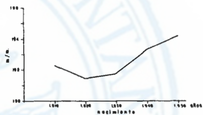
Fig. 4 Longitud Cefálica máxima
