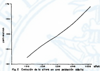
Fig. 2 Evolución de la altura en una población adulta
