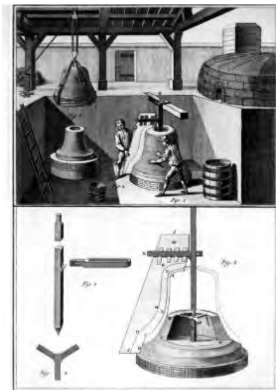
Fundición de una campana, ilustración de L'Encyclopédie ou Dictionnaire raisonné des sciences, des arts et des métiers, enciclopedia francesa editada entre los años 1751 y 1772, bajo la dirección de Denis Diderot y Jean d'Alembert.
